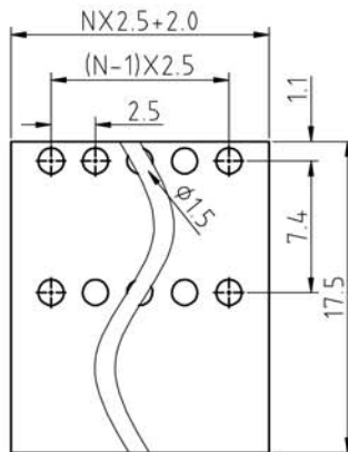
P.C.B. LAYOUT
